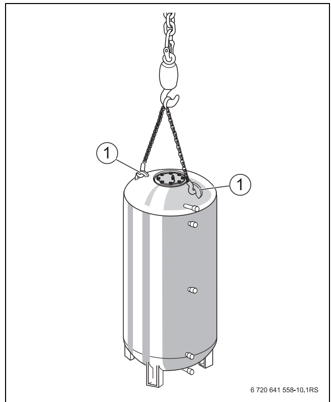
Рис. 5 Подъём краном
